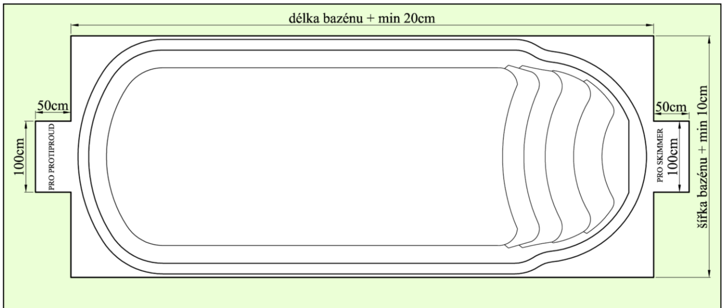
Grabengrundriss
